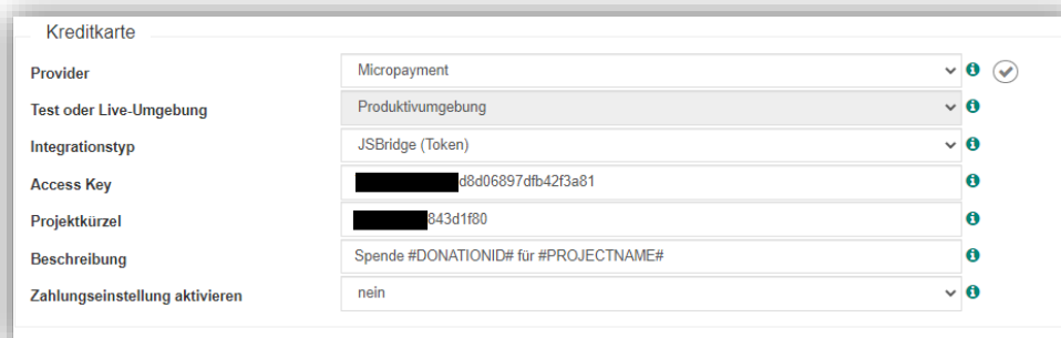
Abbildung 7: Access Key
