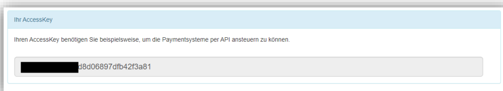
Abbildung 6: Access Key
